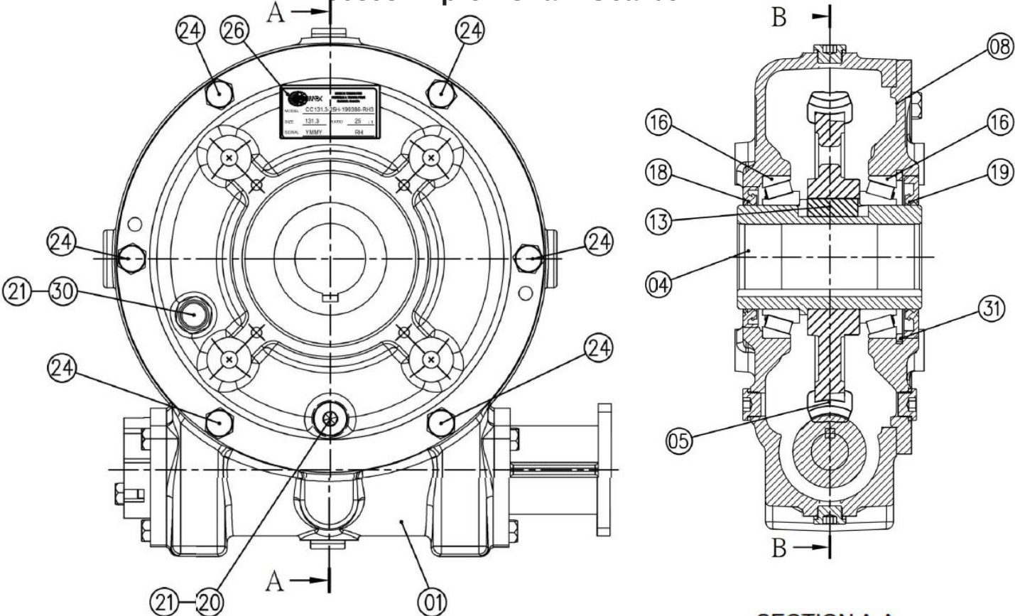
SECTION A-A
